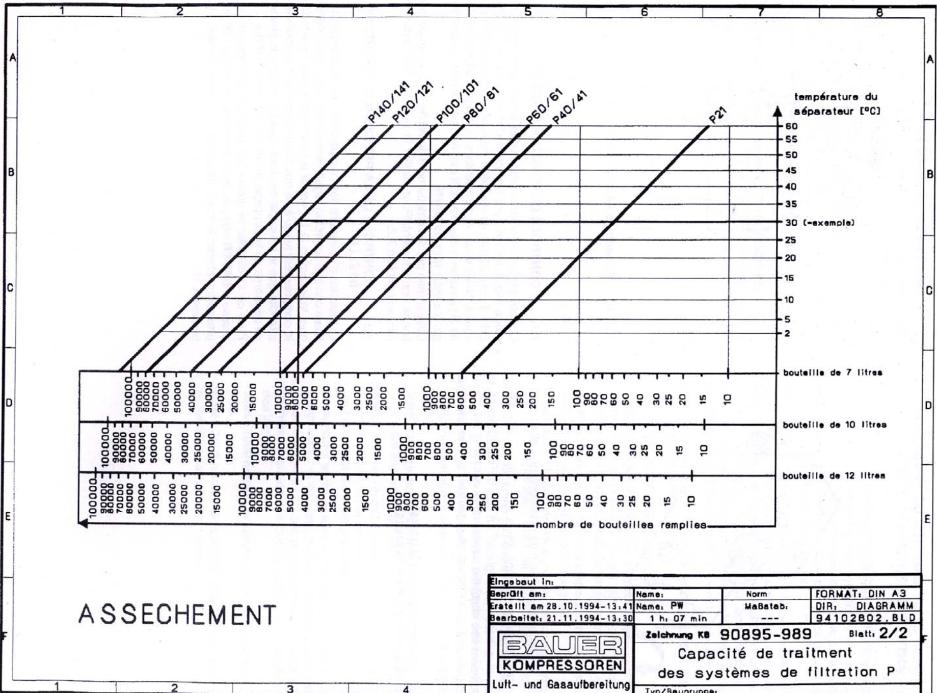
Fig. 12 Capacité de traitement des systèmes de filtration P (feuille 2/2)
