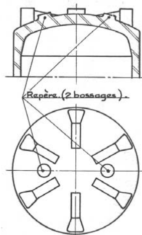
Figure 1 : aspect des 2 bossages sur les fond à pieds
