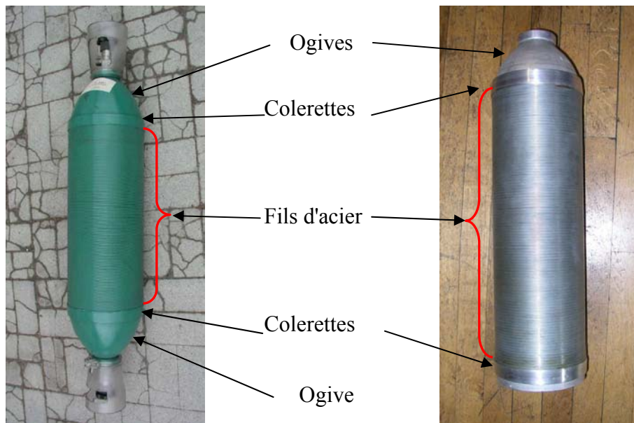
Figure 5 : bouteille frettée fil d'acier 2 ogives
